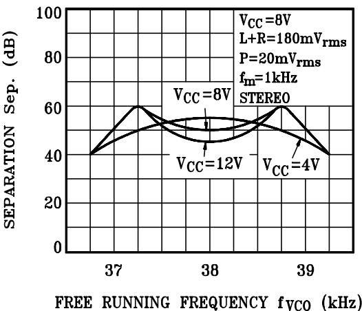
Sep. - f_{VCO}
